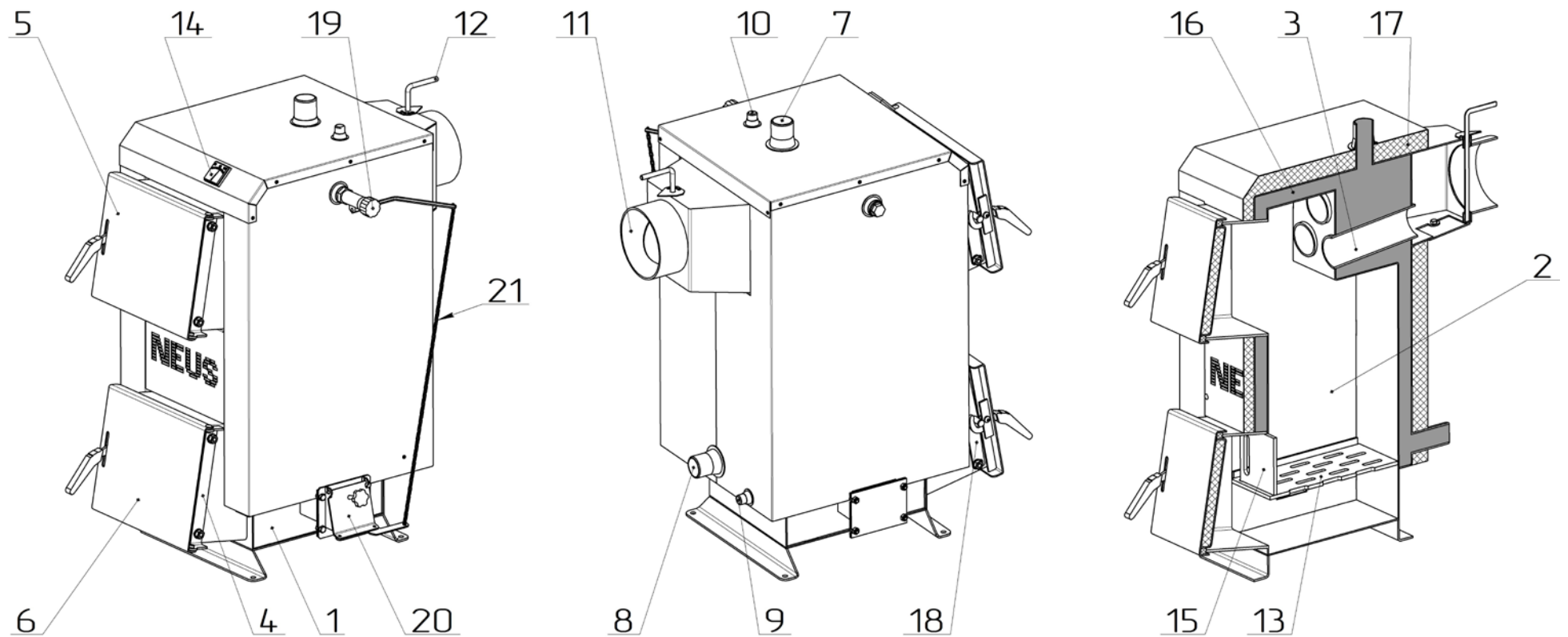
Рисунок 2а – Основні елементи котла Неус-Економ
