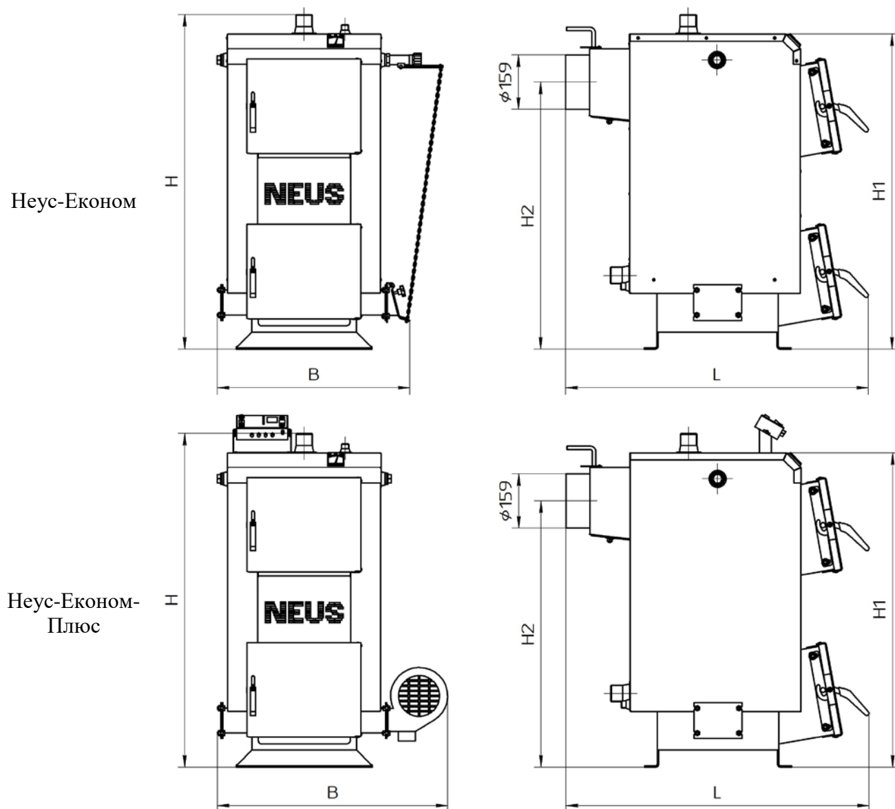
Рисунок 1 – Габаритне креслення котла Неус-Економ (Неус-Економ-Плюс)
