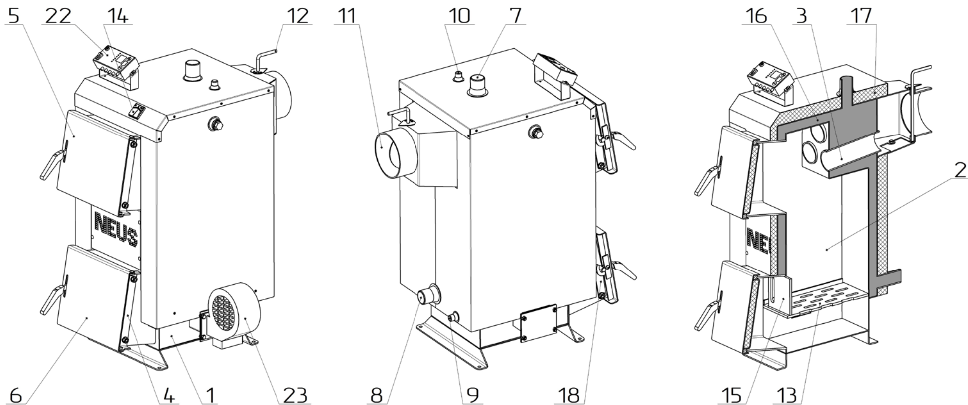
Рисунок 26 – Основні елементи котла Неус-Економ-Плюс
